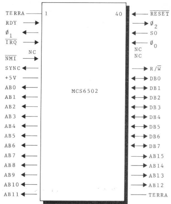
Figura 2 — Pinagem do microprocessador 6502
